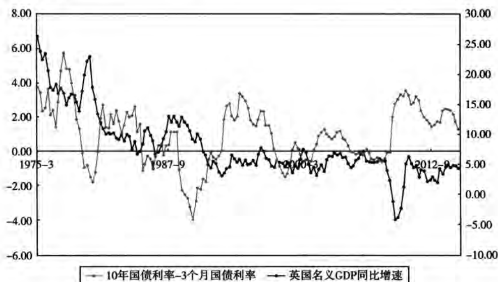
图 3-2-5 英国国债利差（10 年国债利率 - 3 个月国债利率） 曲线与英国名义 GDP 长周期的关系
