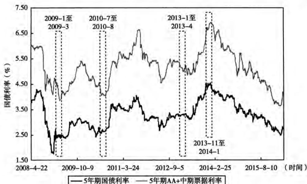
图 7-1-3 信用债券利率与国债利率趋势相关，短暂时期内出现过背离
