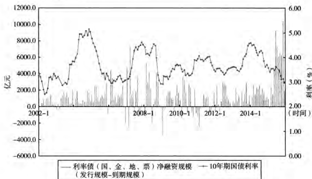
图 1-5-8 2002~2015 年以来债券的净融资规模与利率方向并无正相关性
